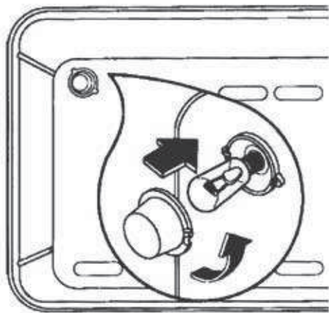
Рис. 11. Замена лампы
