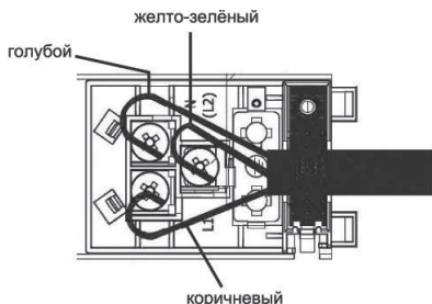
Рис. 10. Схема подключения
