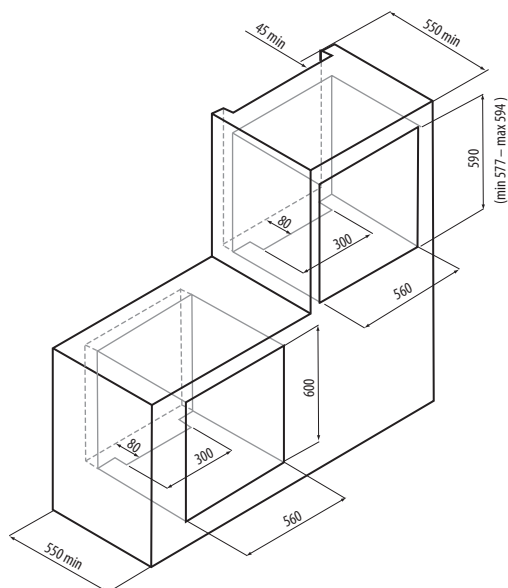
Рис. 8. Схема встраивания духового шкафа
