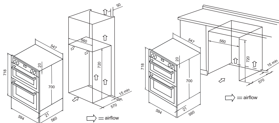
Рис. 6. Схема встраивания духового шкафа
